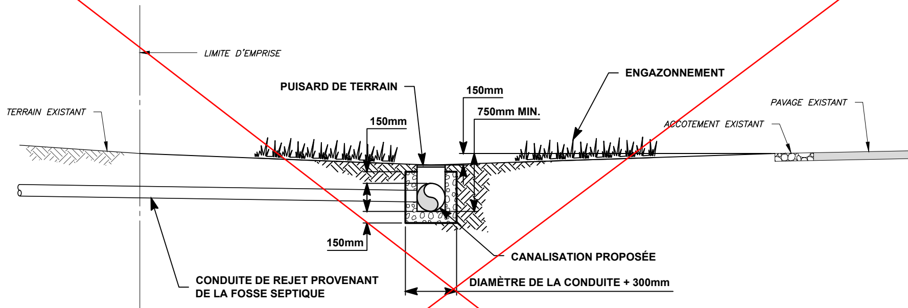
COUPE A-A
